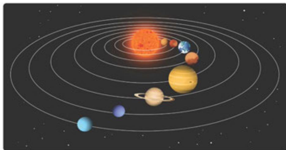
Рисунок 14. Солнечная система
