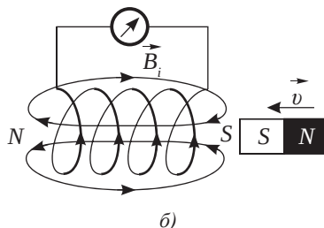
Рис. 324. Индукционный ток на конце катушки, обращенном к приближающемуся магниту, создает одноименный полюс
