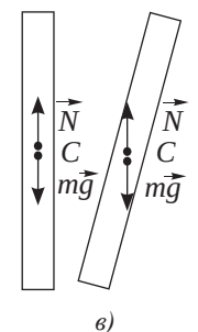
Рис. 61. Равновесие тела на оси вращения
