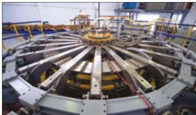
Рис. 296. Казахстанский термоядерный материаловедческий проект «Токамак», запущен в ВКО в день открытия выставки ЭКСПО-2017
