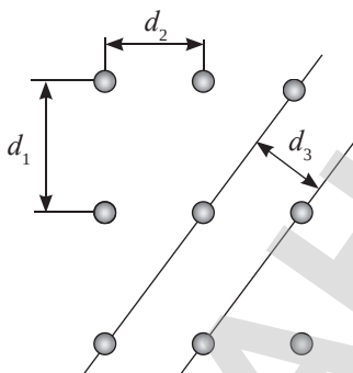
Рис. 140. Монокристаллы анизотропны
