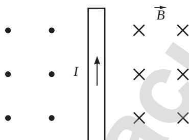
Рис. 271. Изображение силовых линий при продольном сечении проводника
