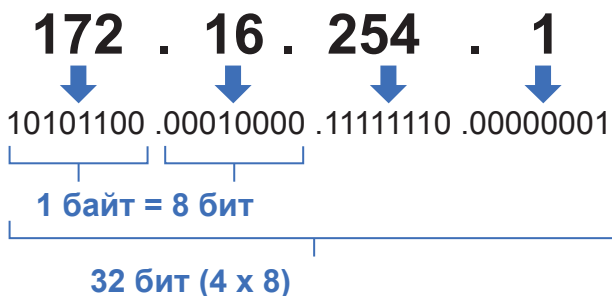
Рис. 4. Пример IP-адреса
