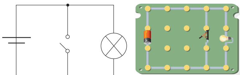
Рис. 9. Электрическая схема логического элемента «HE»
