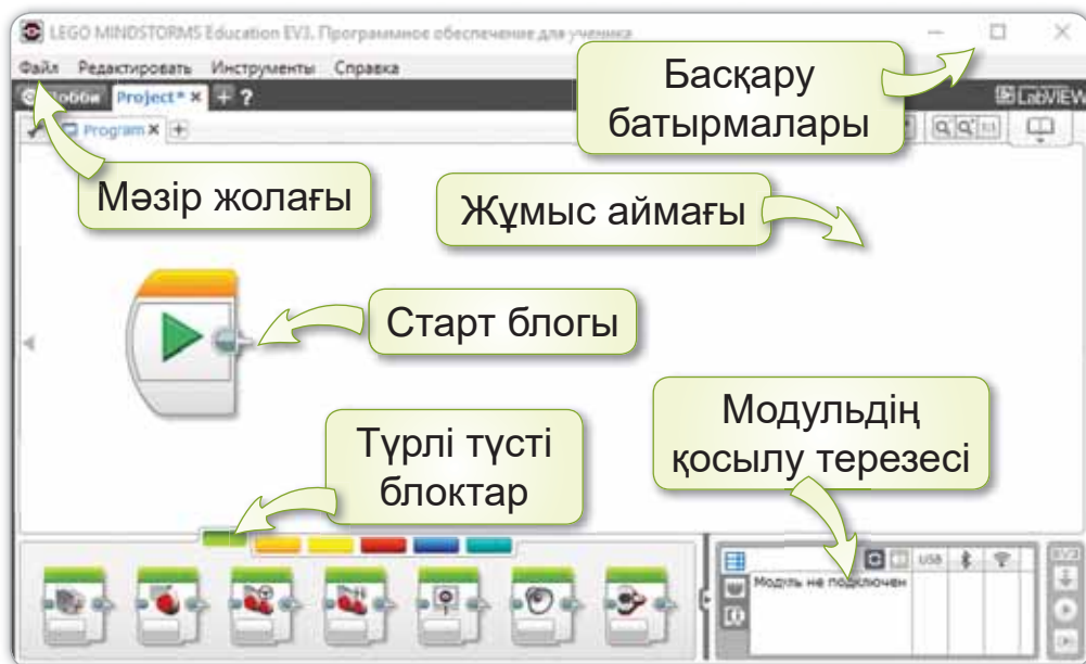
35-сурет. LME EV3 программасының жұмыс аймағы
