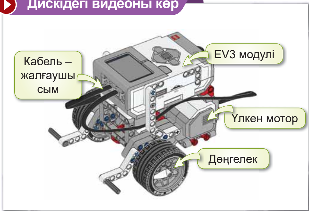
29-сурет. Білім беру роботы
