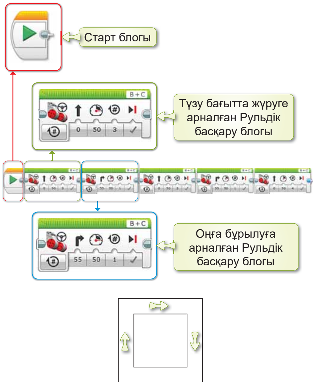
57-сурет. Программа нәтижесі
